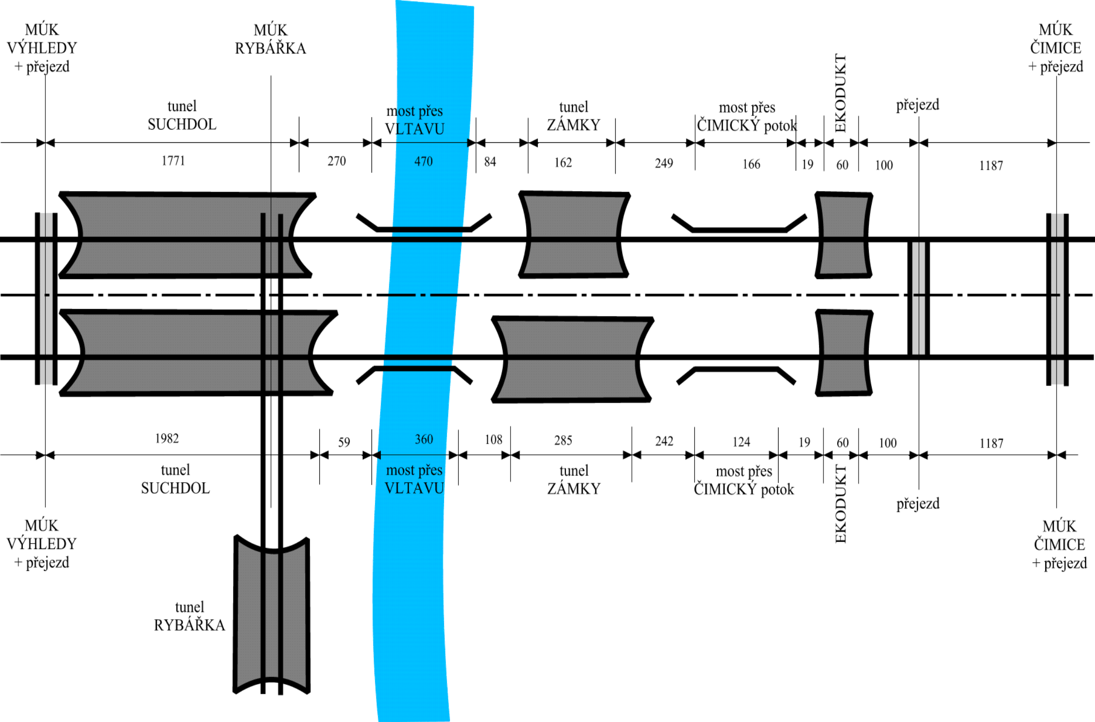
Liniové schéma části trasy staveb 518 a 519 tvořící jeden úsek z hlediska bezpečnosti provozu
